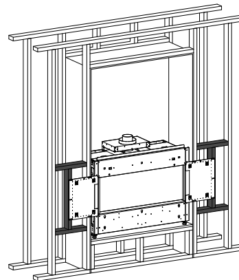
8-1/2 po du centre d'un montant à l'autre
