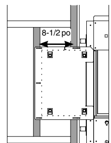
8-1/2 po du centre d'un montant à l'autre
